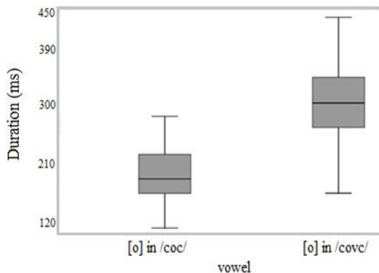
شکل (۵): نمودار جعبه‌ای دیرش واکه [o] در /coc/ و /covc/ برای تمامی شرکت‌کنندگان آزمایش
