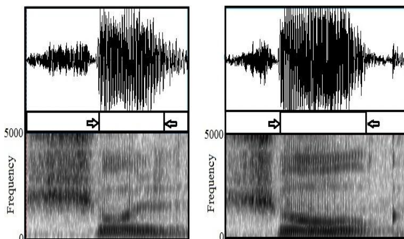
شکل (۱): طیف‌نگاشت کلمات [شل] (چپ) و [شوق] (راست) تولید شده توسط گویشور س. م.
