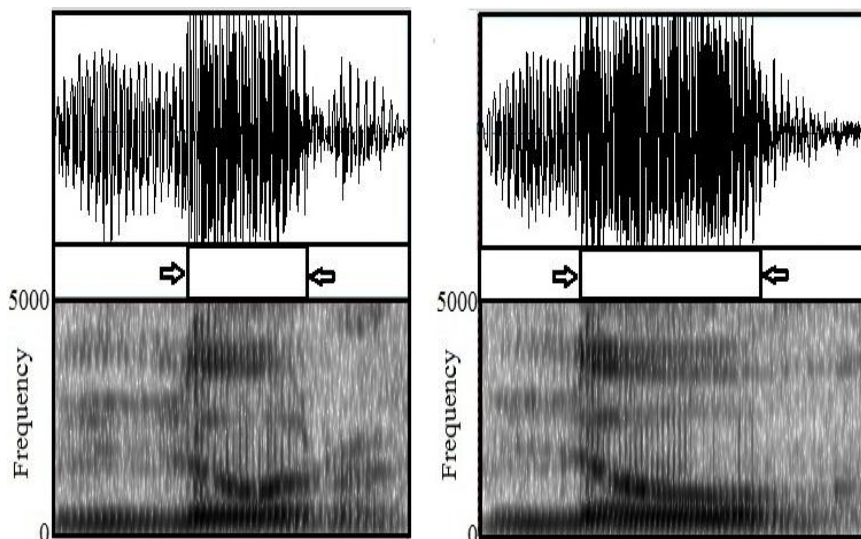
شکل (۲): طیف‌نگاشت کلمات [کَاش] (چپ) و [کَاش] (راست) تولید شده توسط گویشور ق. ک.
